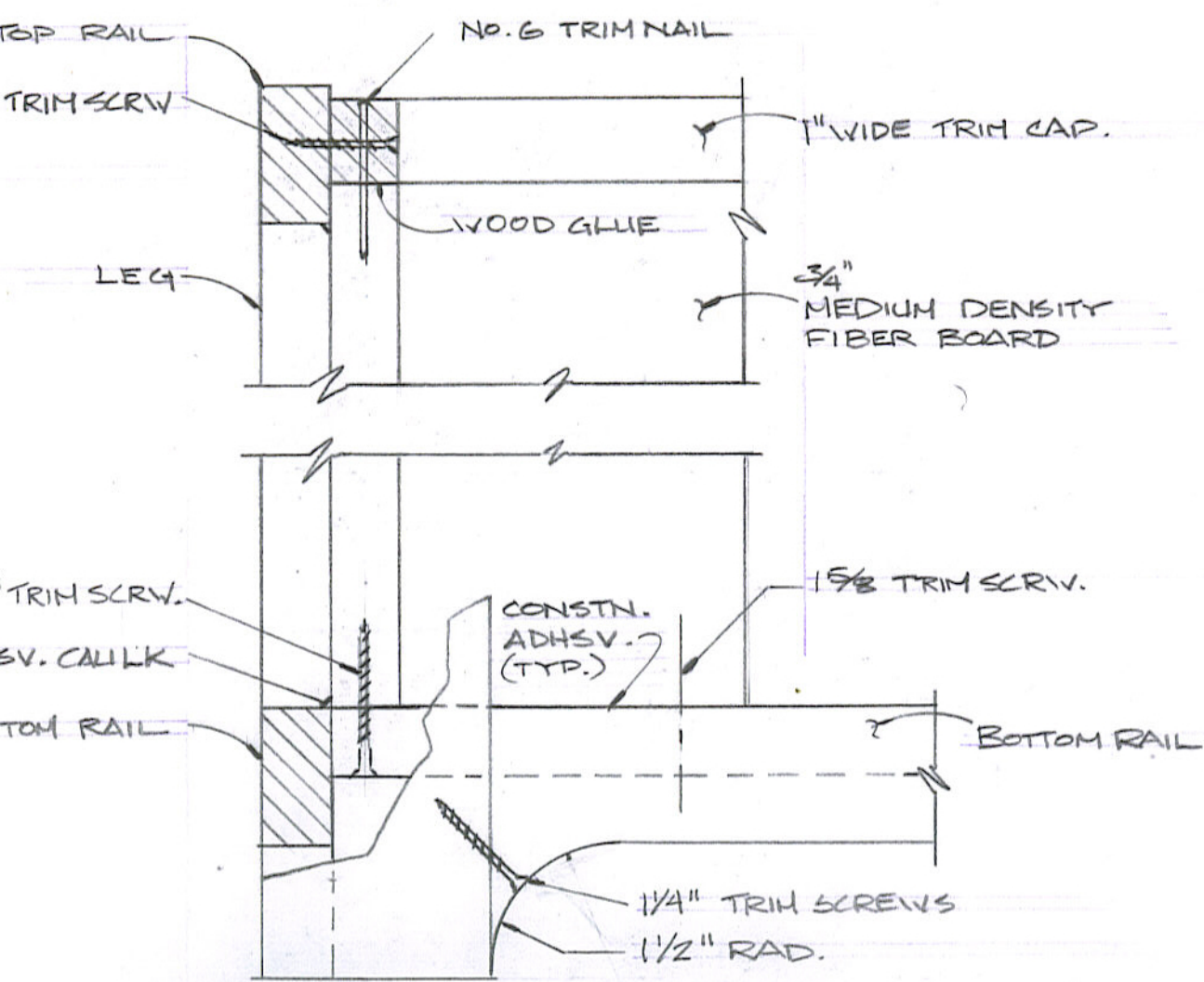
DETAIL A-A
